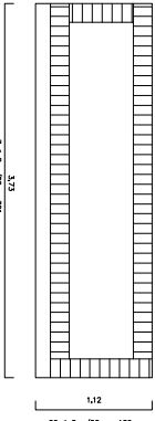
ARMAÇÃO DA LAJE DE FUNDO Escala 1:25
