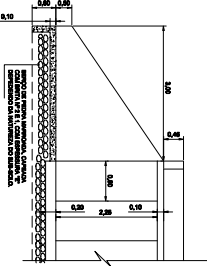
SEÇÃO LONGITUDINAL Escala 1:50
