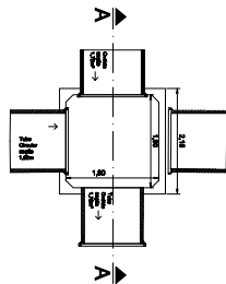
PLANTA BAIXA Escala 1:50
