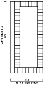
ARMAÇÃO DA LAJE DE FUNDO Escala 1:25
