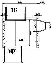
CORTE A-A Escala 1:50
